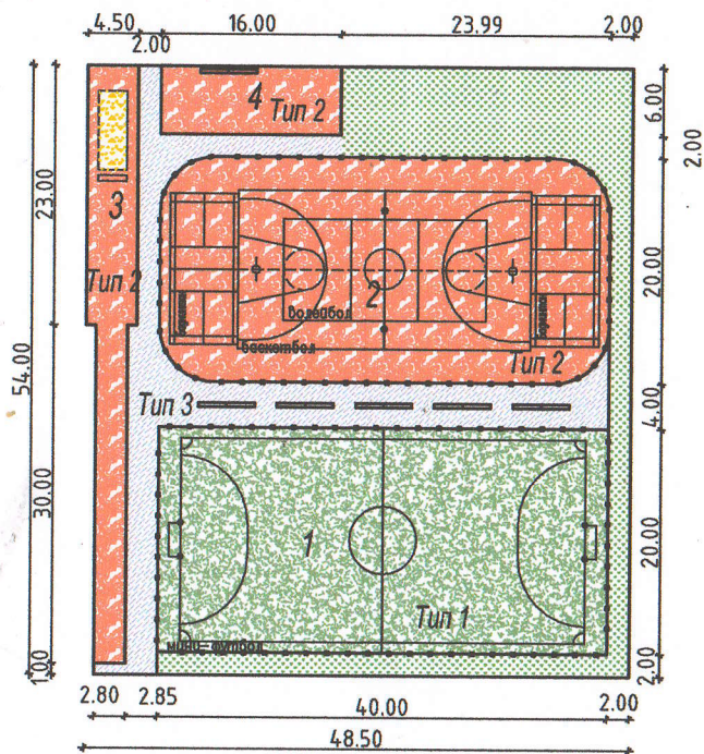
Схема планировочной организации земельного участка. М 1:500
